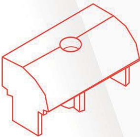
Kanat Kaldırma Takozu (Kanada Montaj) Lifting Wedge for Sash (Mounting to Sash) Фиксатор-балансир створки ترفيعة الضلفة (يركب على الضلفة)
