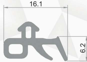
18mm Universal conta Universal Joint for 18 mm 18 мм уплотнитель стекла جوان أوني وارسال ١٨ مم
