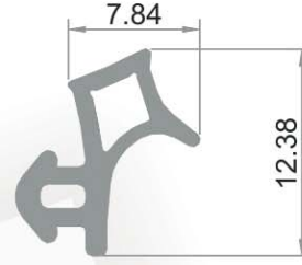
Kasa-kanat contası Frame - Sash Joint уплотнитель рама-створка جوان للإطار والصفافة
